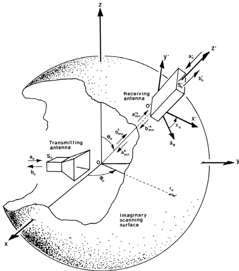
sistema di trasmissione per scansione sferica
