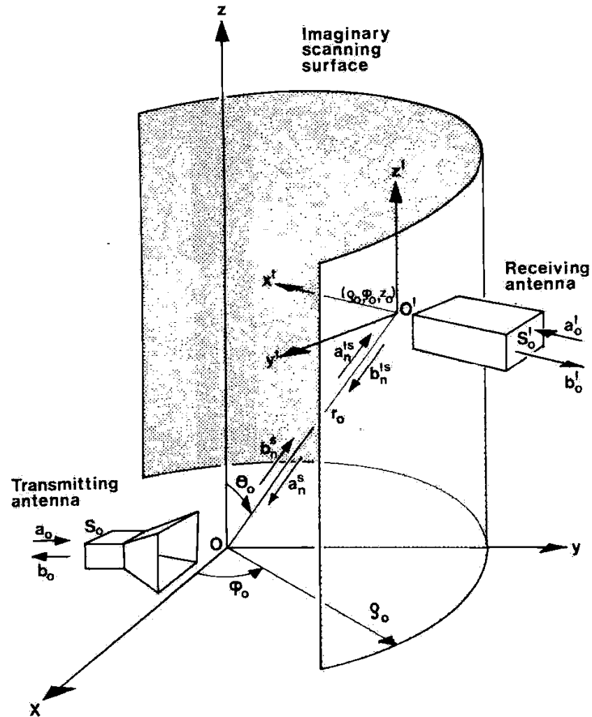
sistema di trasmissione per scansione cilindrica
